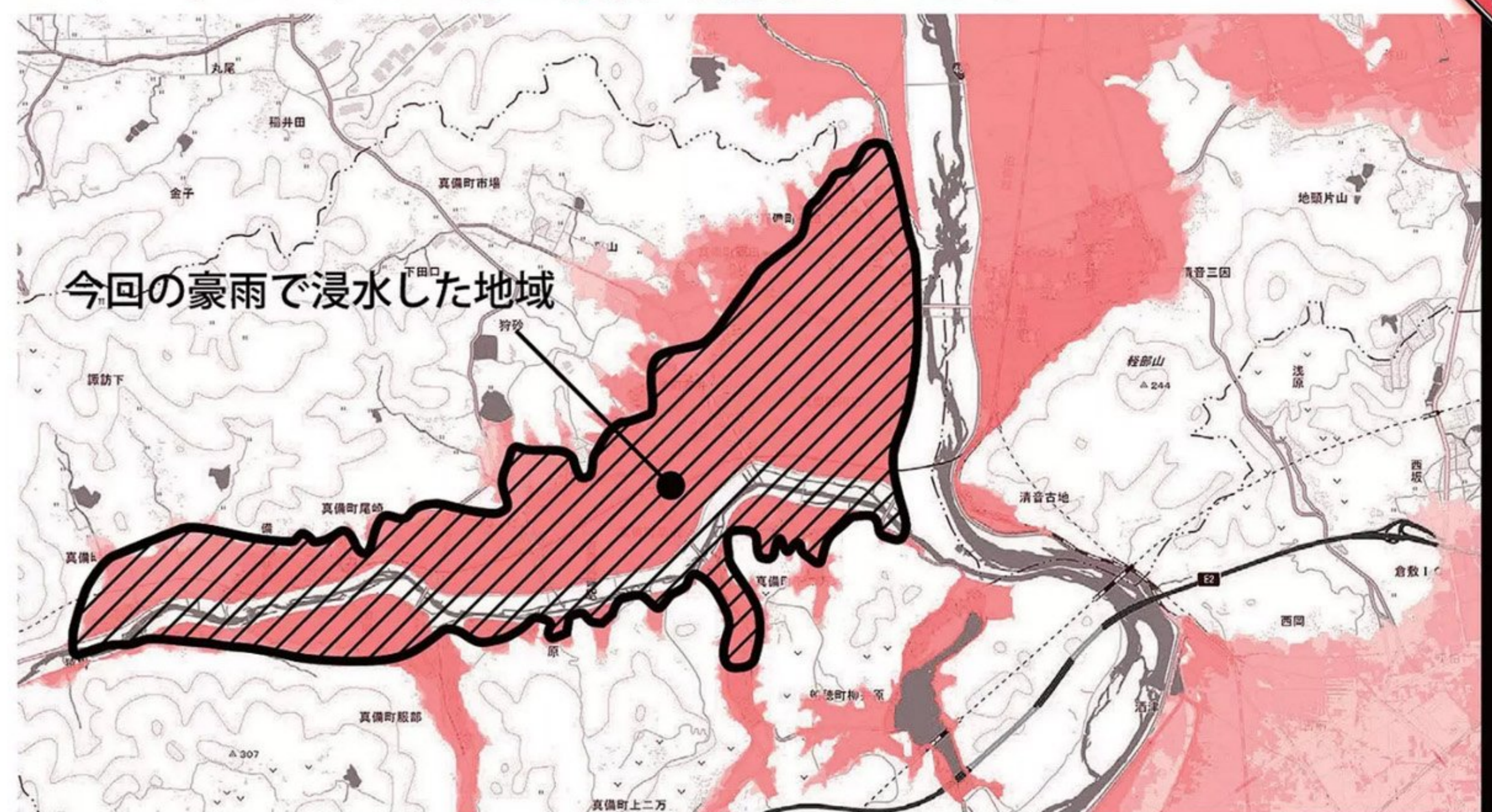
国土交通省「重ねるハザードマップ」で真備町の「洪水浸水想定区域」を表示すると、今回の浸水域とほぼ一致している。想定される浸水の深さは10m以上となっており、洪水リスクが非常に高い地域だったことがわかる。「重ねる～」では土砂災害、津波のリスク情報や、道路防災情報、土地の成り立ちなども表示できる
