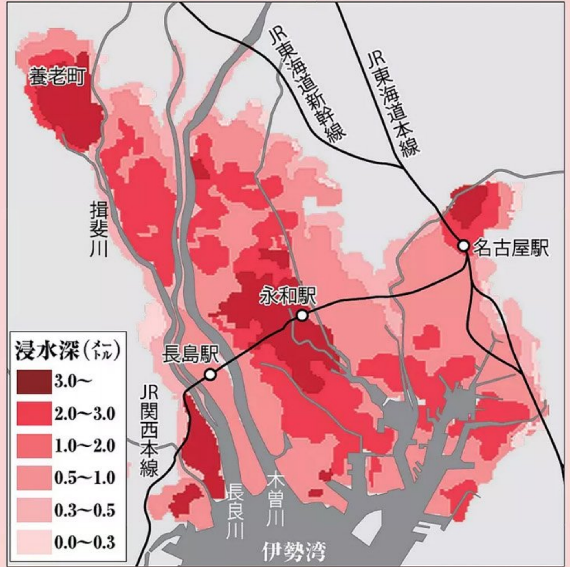
明治以降で最大の被害を出した伊勢湾台風。広い範囲で高潮が発生、急速な工業発展にともなう地盤沈下が原因で愛知県では3千人以上の犠牲者が出た
